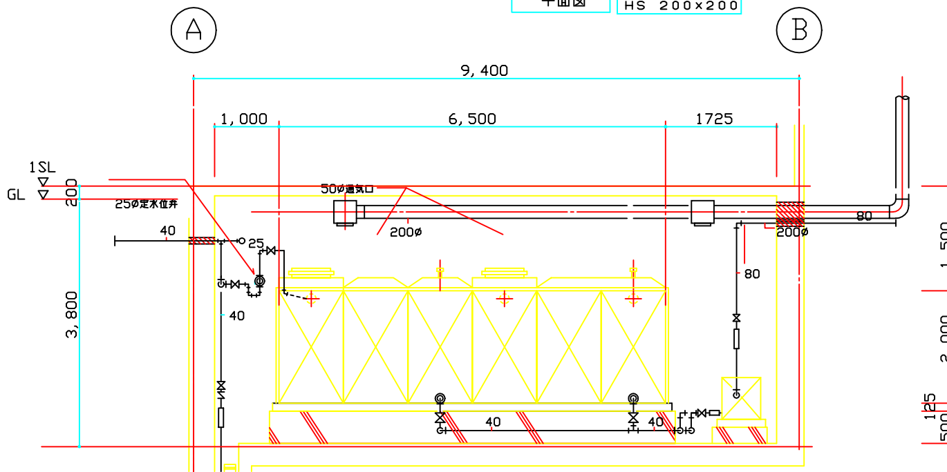
平面図 吹出口 HS 200×200
