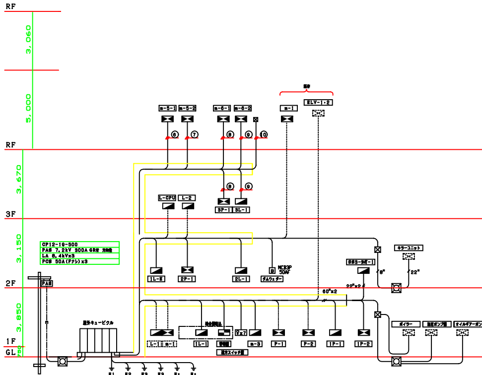
設備系統図 実寸中電線サイズは緑地線を示す。
