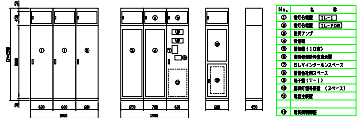
組合器図 実寸法は参考とす。
