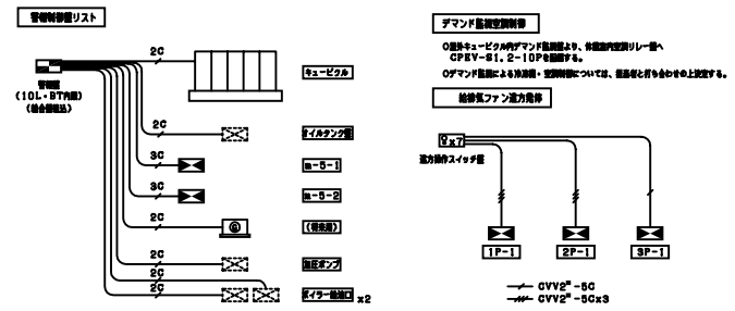
組合器図 実寸法は参考とす。
